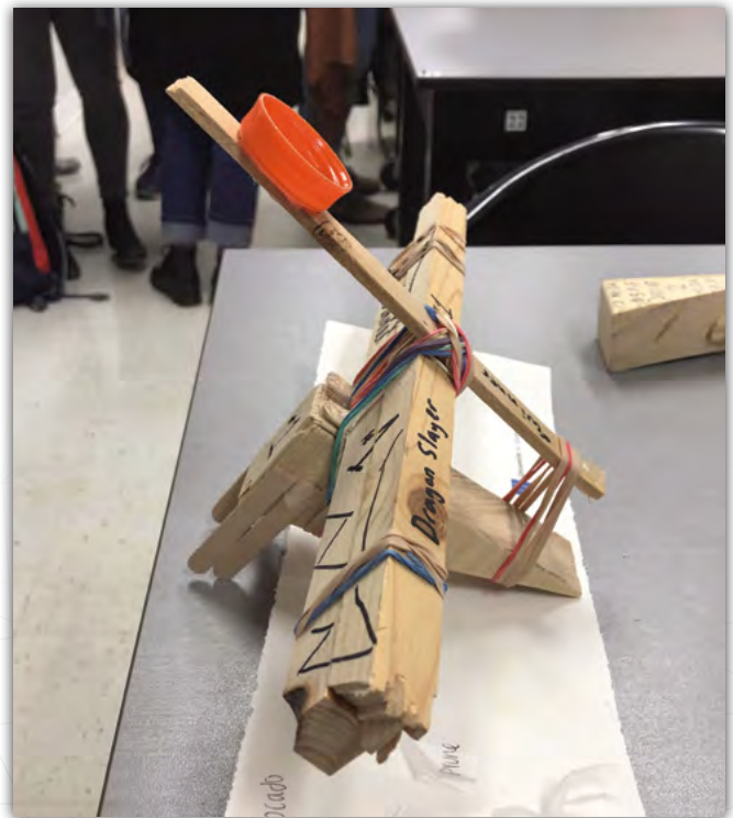
Prototypé de catapulte réalisée par des étudiants universitaires
